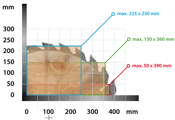
BL 225 Ø 700 mm
