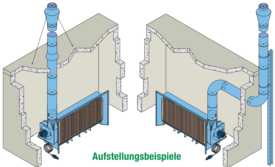
Schuko FarbMax mit Abluftführung durch die Decke
